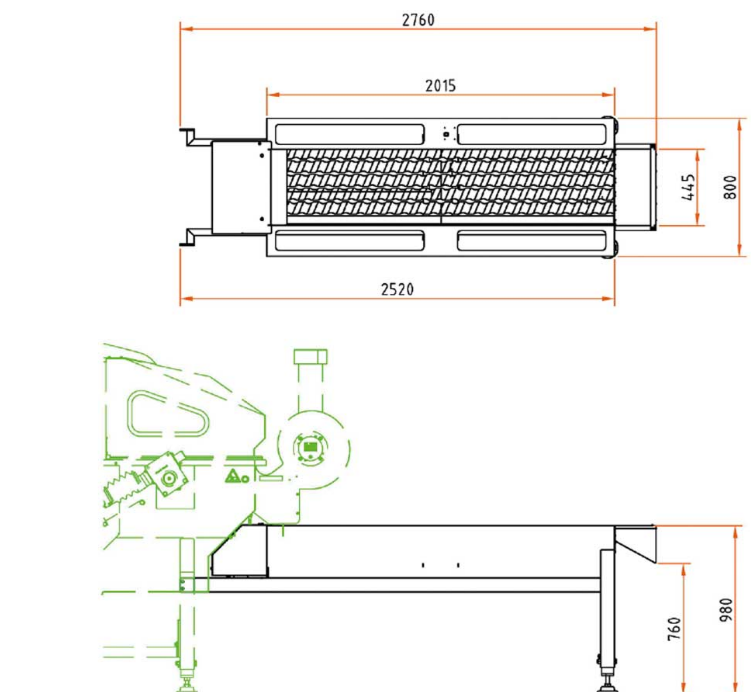
Planos acotados basados en el diseño RLT-L6/200
